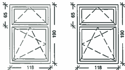
KOLOR OKIEN: ZEWNĘTRNY-BIAŁY, WEWNĘTRZNY-BIAŁY
