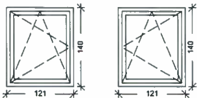
KOLOR OKIEN: ZEWNĘTRNY-BIAŁY, WEWNĘTRZNY-BIAŁY
