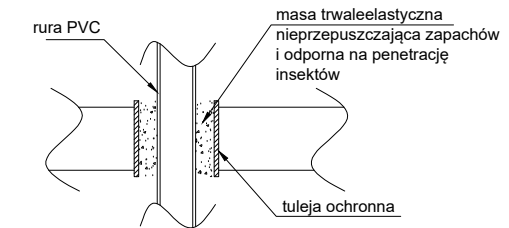
Detal przejścia rury przez przegrody budowlane
